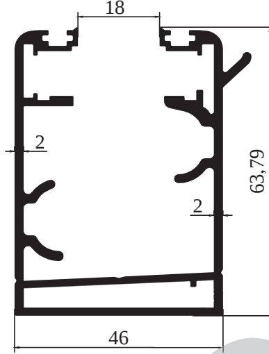
M 2152 - 1,626 kg/m
