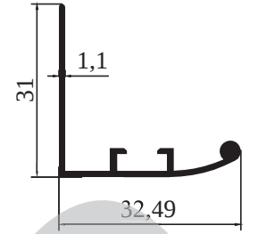
1130 - 0,250 kg/m
