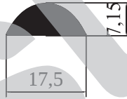
8555 - 0,244 kg/m
