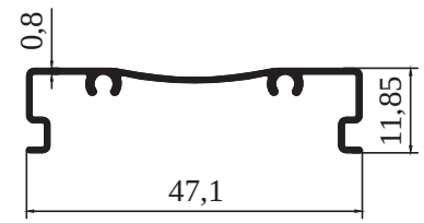
8392 - 0,207 kg/m
