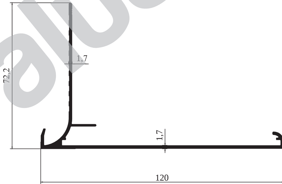
M 8549 - 1,017 kg/m
