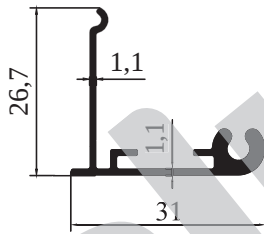
8230 - 0,290 kg/m
