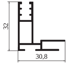
9153 - 0,369 kg/m
