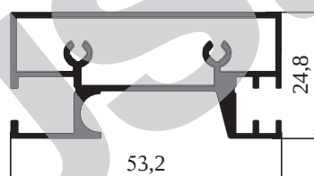
9091 - 0,731 kg/m STOK BOY : 6,00 cm
