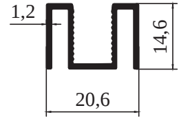
M 2399 - 0,235 kg/m
