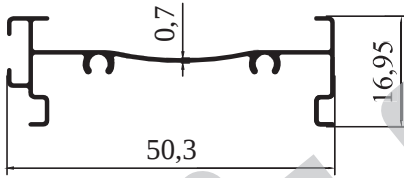
8013 - 0,234 kg/m
