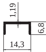
M 1528 - 0,341 kg/m
