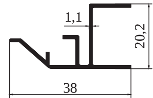
8553 - 0,263 kg/m
