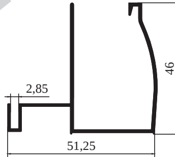
4126 - 0,506 kg/m STOK BOY : 5,80 cm
