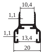
M 2135 - 0,240 kg/m
