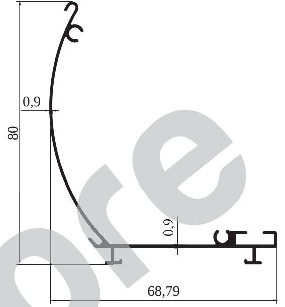
8458 - 0,502 kg/m
