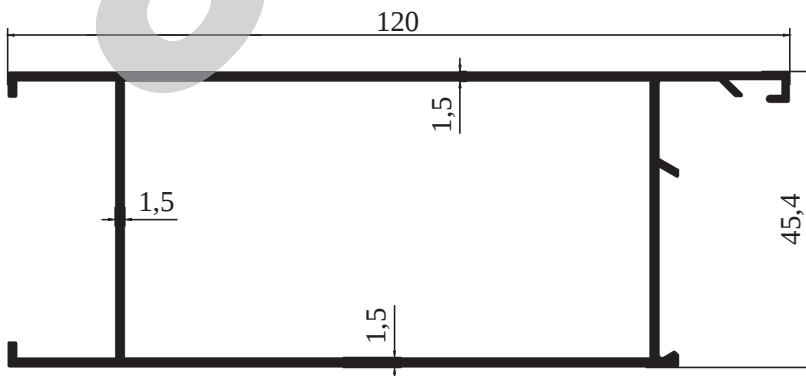
M 3010 - 1.312 kg/m
