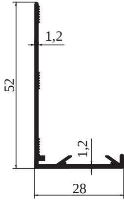
1143 - 0,309 kg/m
