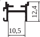
M 2204 - 0,155 kg/m
