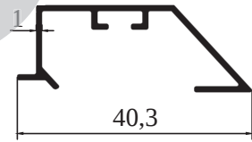
M 9509 - 0,219 kg/m
