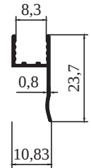
M 938 - 0,097 kg/m
