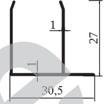
4453 - 0,222 kg/m STOK BOY : 5,80 cm
