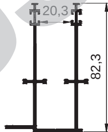
M 2406 - 1.290 kg/m
