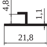
8900 - 0,094 kg/m
