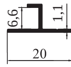
M 8053 - 0,092 kg/m
