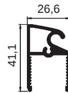
M 2467 - 0.673 kg/m
