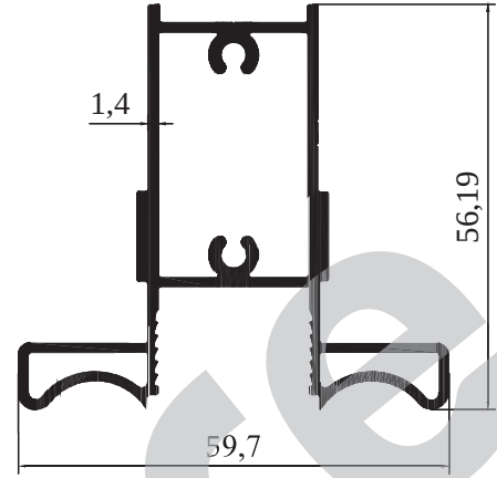
M 2309 - 1,113 kg/m
