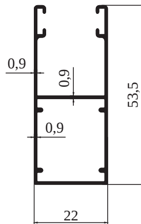
8427 - 0,420 kg/m
