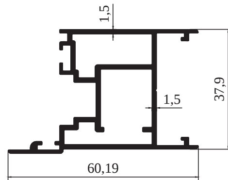
M 2157 - 0,954 kg/m
