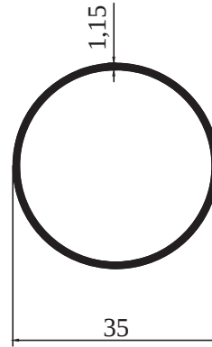
M 1528 - 0,341 kg/m
