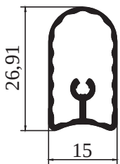
8014 - 0,243 kg/m
