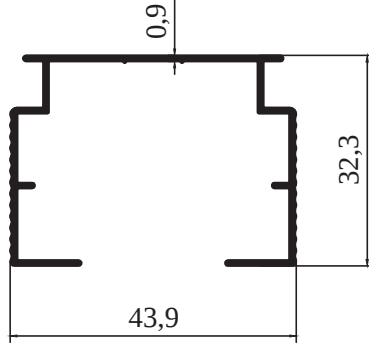
8437 - 0,347 kg/m
