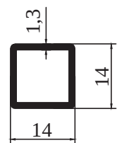
M 1416 - 0,151 kg/m
