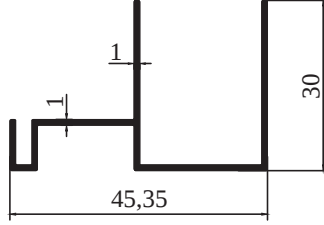
4143 - 0,325 kg/m STOK BOY : 5,80 cm
