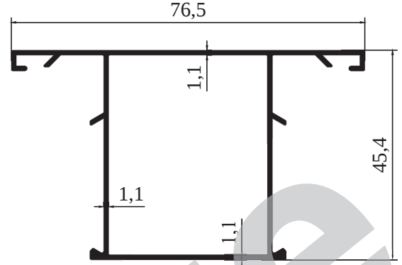
M 3006 - 0,706 kg/m
