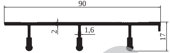
M 9501 - 0,799 kg/m
