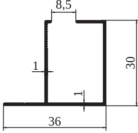
4142 - 0,279 kg/m STOK BOY : 5,80 cm
