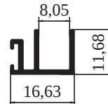
M 2207 - 0,159 kg/m
