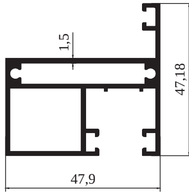
M 2054 - 0,962 kg/m
