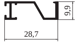
8611 - 0,185 kg/m
