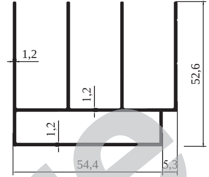
M 2211 - 0,949 kg/m
