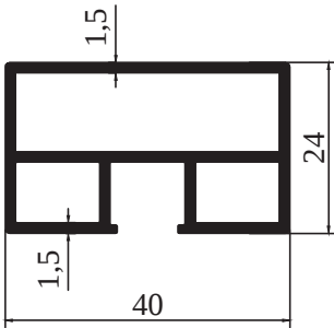
M 2055 - 0,678 kg/m
