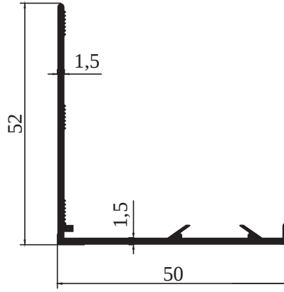
1144 - 0,464 kg/m
