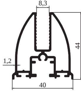
M 2112 - 0,840 kg/m
