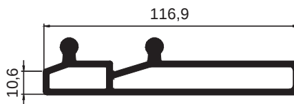
M 2495 - 1.777 kg/m
