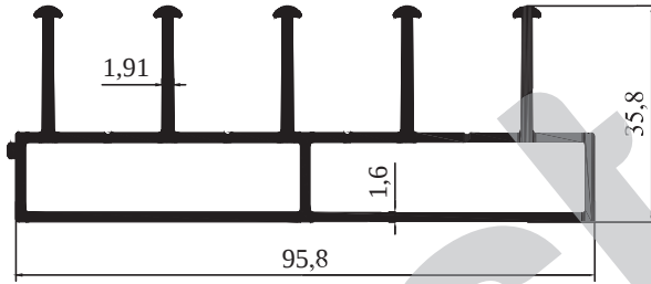
M 2202 - 1,567 kg/m
