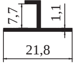
8899 - 0,104 kg/m
