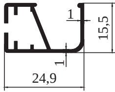
8532 - 0,222 kg/m
