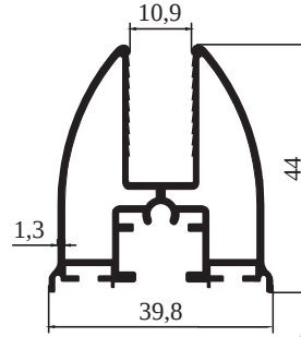
M 2113 - 0,850 kg/m
