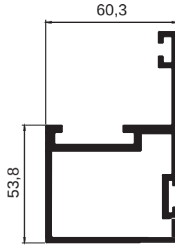
M 2461 - 0.585 kg/m
