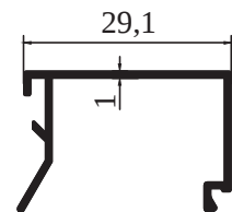
M 3020 - 0.210 kg/m
