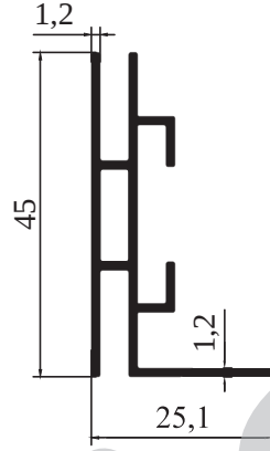
M 9202 - 0,588 kg/m
