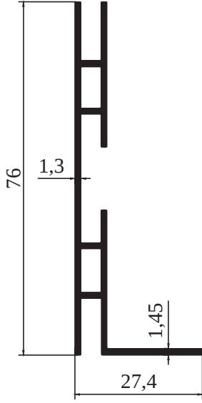
M 9521 - 0,629 kg/m
