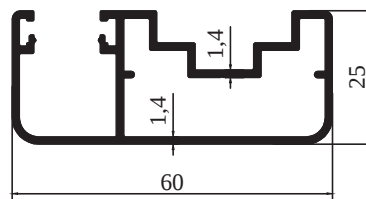
M 2071 - 0,781 kg/m
