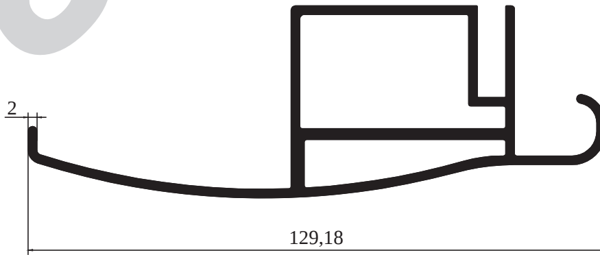
M 2373 - 1,917 kg/m
