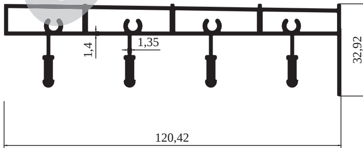
M 2362 - 1,911 kg/m
