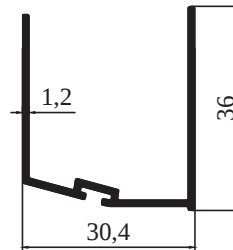
4135 - 0,328 kg/m STOK BOY : 5,80 cm
