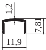
M 2011 - 0,642 kg/m
