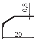
9033- 0,054 kg/m
