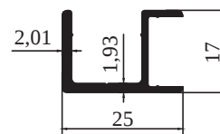
M 9532 - 0,276 kg/m
