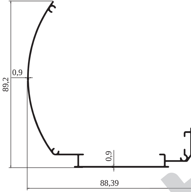
8131 - 0,543 kg/m
