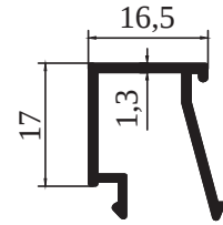
M 3112 - 0.225 kg/m
