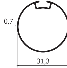
5556 - 0,205 kg/m
