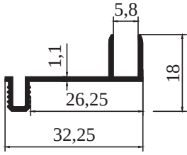
8052 - 0,193 kg/m STOK BOY : 6,00 cm
