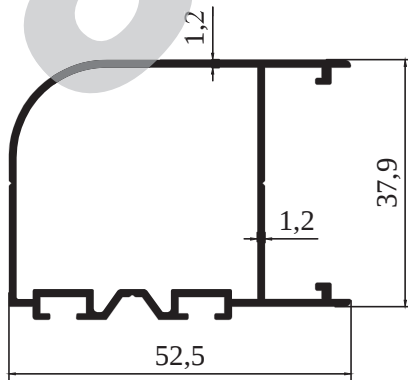
M 2156 - 0,648 kg/m
