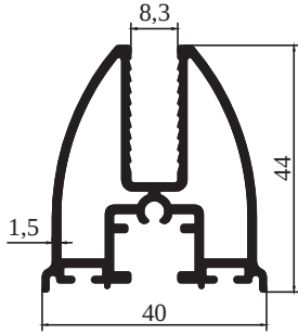
M 2111 - 0,898 kg/m
