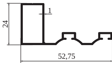
3814 - 0,359 kg/m STOK BOY : 5,40 cm
