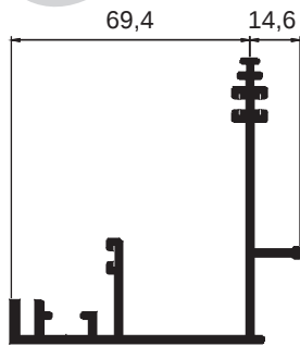
M 2494 - 1.151 kg/m
