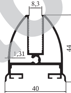
8194 - 0,837 kg/m
