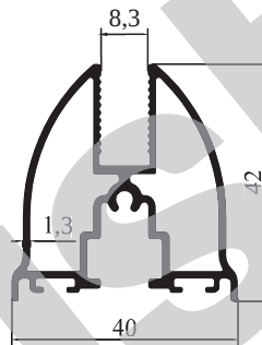
8444 - 0,816 kg/m
