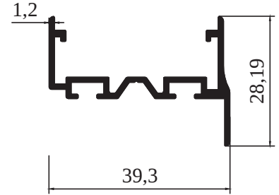
M 2155 - 0,374 kg/m
