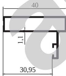
M 2121 - 0,376 kg/m
