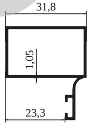
M 2123 - 0,365 kg/m
