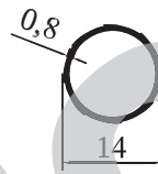
8416 - 0,098 kg/m
