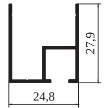
9090 - 0,280 kg/m STOK BOY : 6,00 cm
