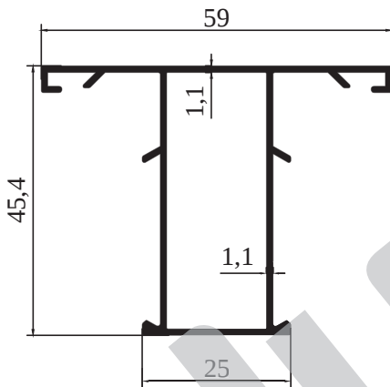
M 3003 - 0,589kg/m
