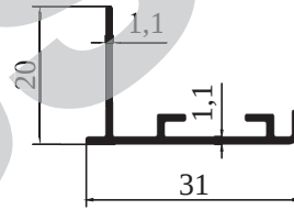
8472 - 0,197 kg/m
