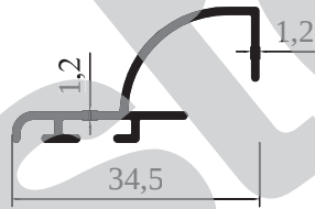
1950 - 0,244 kg/m
