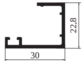
M 2050 - 0,308 kg/m
